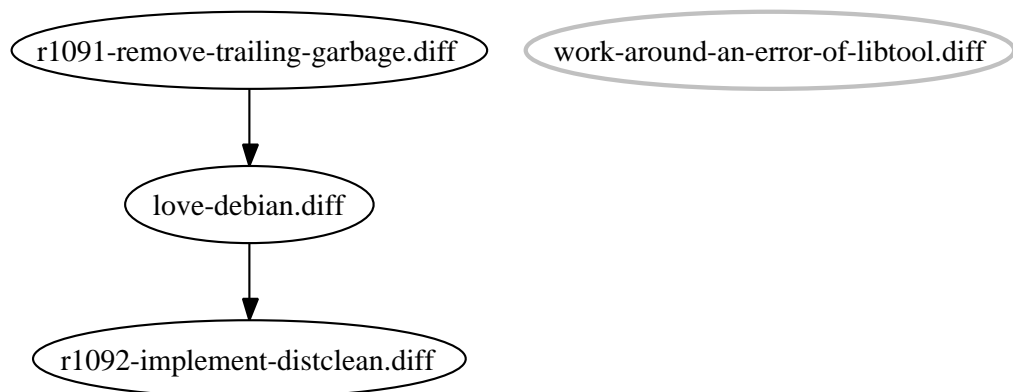
図 2 変更領域が 1 行被っている場合に依存関係がある、として計算した依存関係
